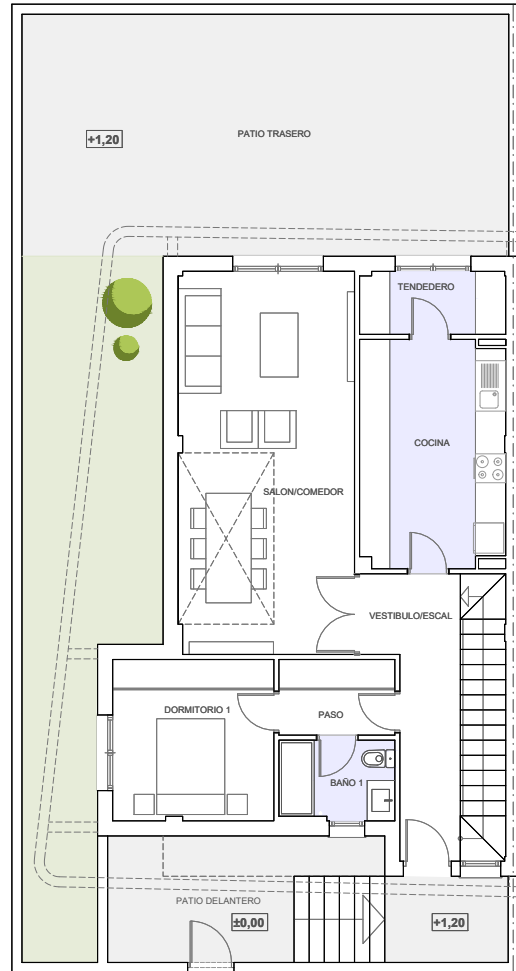
PLANTA BAJA
