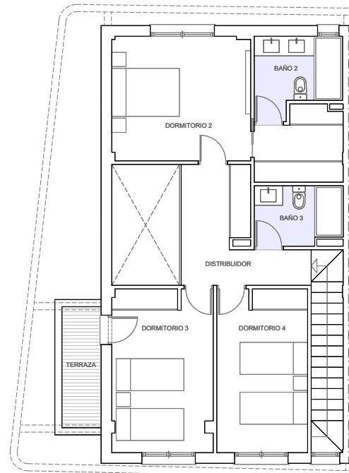
PLANTA PRIMERA
