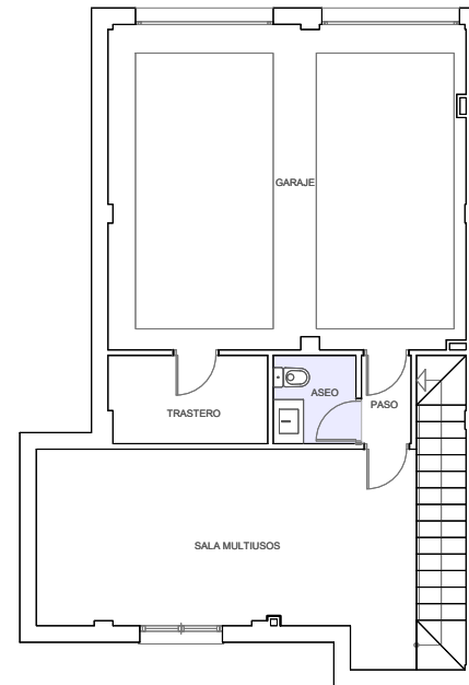
PLANTA GARAJE
